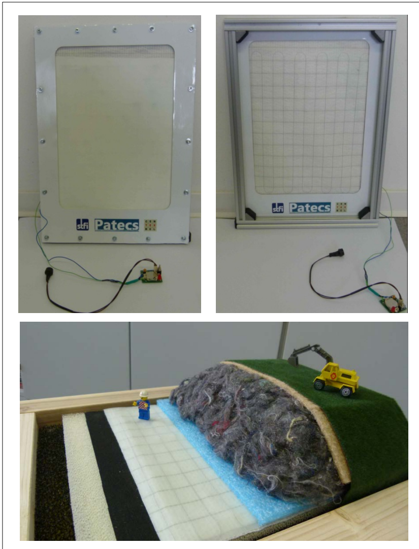
Abb. 3: Entwickelte Demonstratoren (Oben: schnittsichere Plane mit Sensorfunktion; Unten: Modell Dichtigkeitsüberwachung einer Deponie)
