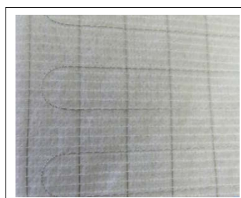
Abb. 2: Integration der Sensormaterialien in die textile Fläche mit Hilfe des Webens und Verbundwirkens
