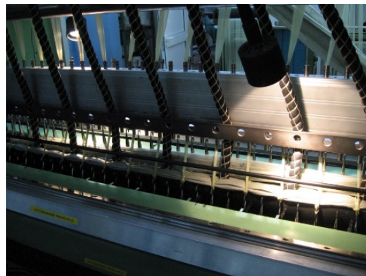
Abb. 1: Zuführung von gefassten Vliesstoffbändern in die Nadelgassen
